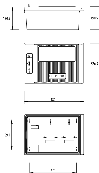
06C2CM Caixas para dois contadores monofásicos
